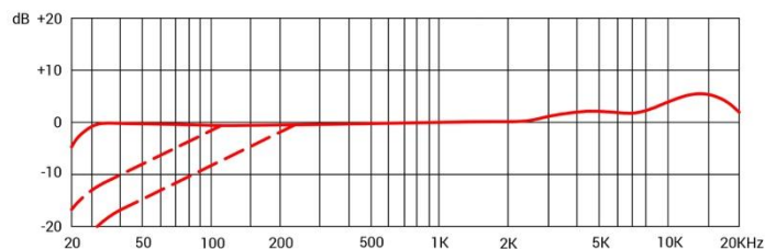
Частотный диапазон
