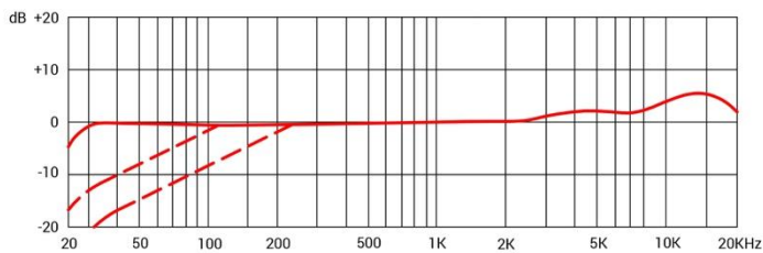
频率响应
