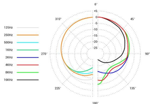
Диаграмма направленности
