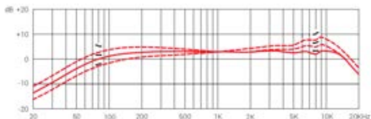
频率响应
