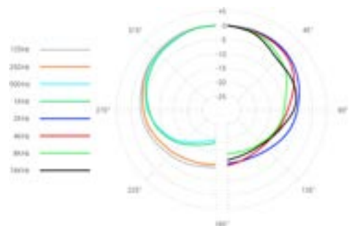
Polardiagramm
