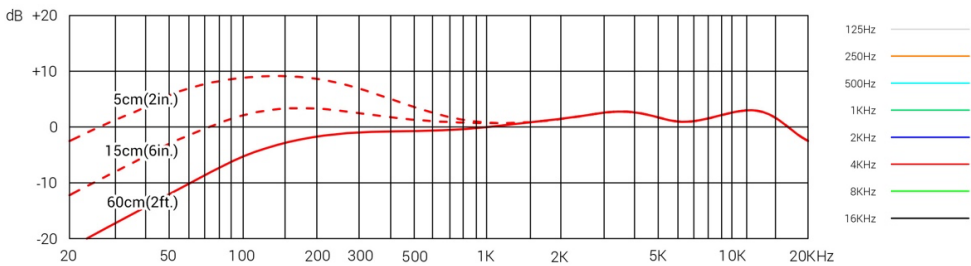
Частотная характеристика
