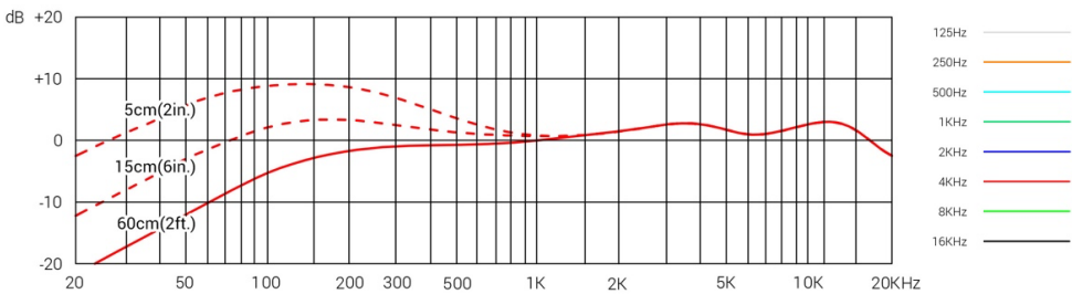
Risposta in frequenza
