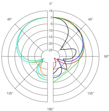
Диаграмма направленности
