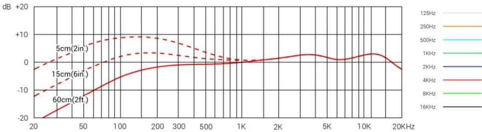
频率响应
