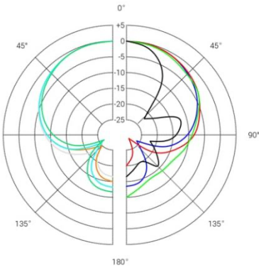
指向性
