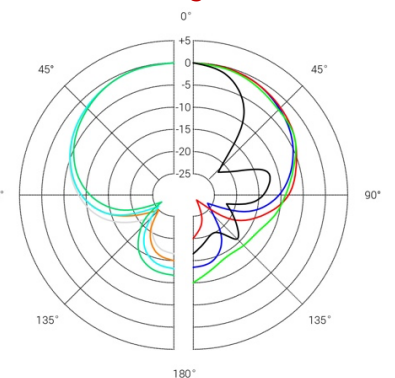
Polardiagramm
