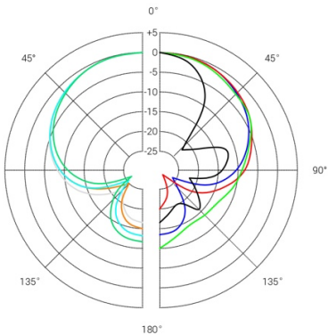
Modèle polaire
