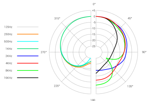
Polaridiagramm
